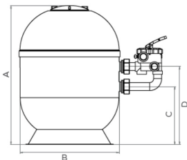
Dimensions d400 - d900
